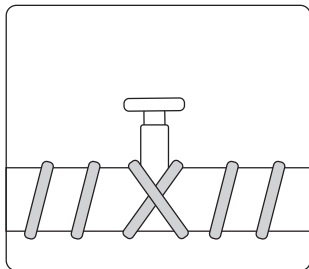
Спиральный монтаж кабеля на трубу
