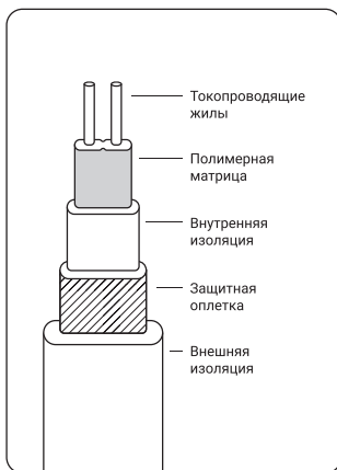
Строение кабеля IN ECO 10
