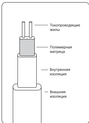
Строение кабеля ON ECO 16
